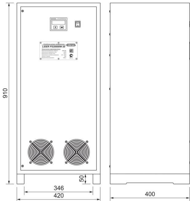
Габаритные и установочные размеры стабилизатора напряжения переменного тока LIDER 2000W – +50/-30
