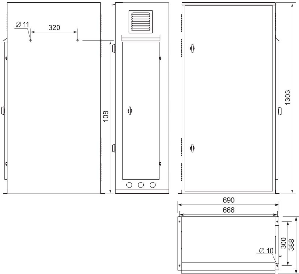
Рисунок 1- Габаритные и установочные размеры шкафа
