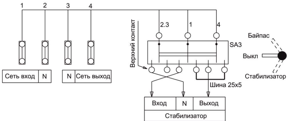
Рисунок 1 – Схема подключения байпаса однофазного ручного
