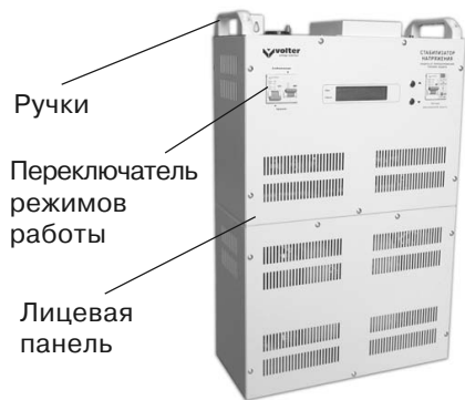
Рис. 1. Стабилизатор напряжения
