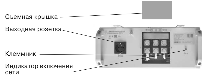
Рис. 5. Верхняя панель стабилизатора
