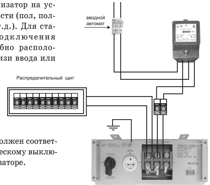
Рис. 10. Схема установки стабилизатора
