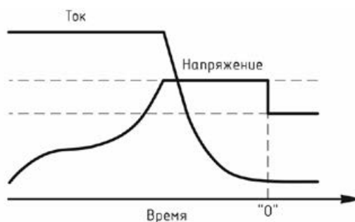
Рис. 6 - Зависимость тока и напряжения от времени при заряде по методу IUoU
